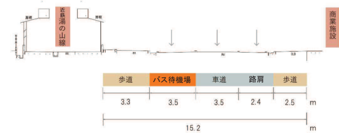
【整備後】
