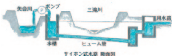
サイホン式水路 断面図
